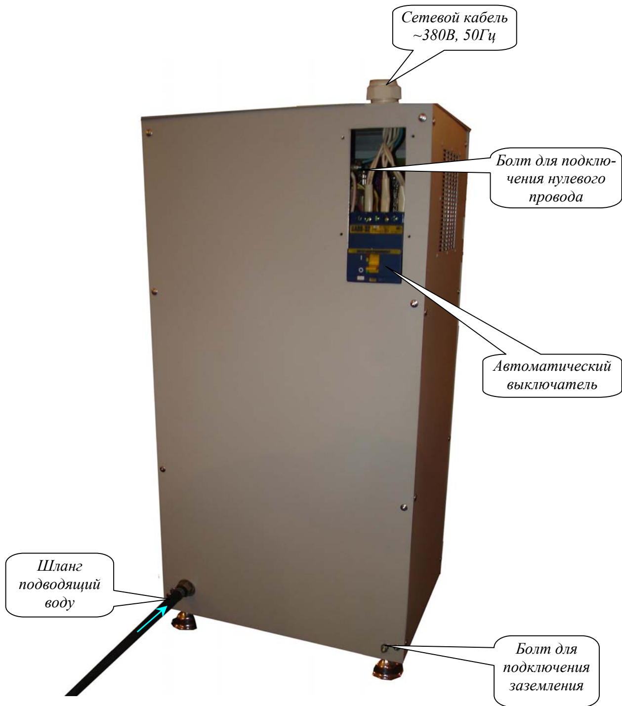
Рисунок 2. Силовой блок преобразователя (задняя панель)
