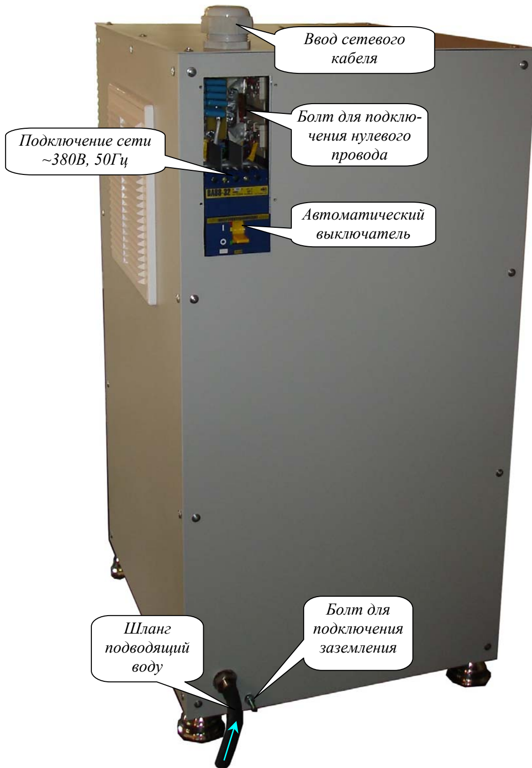
Рисунок 2. Силовой блок преобразователя (задняя панель)
