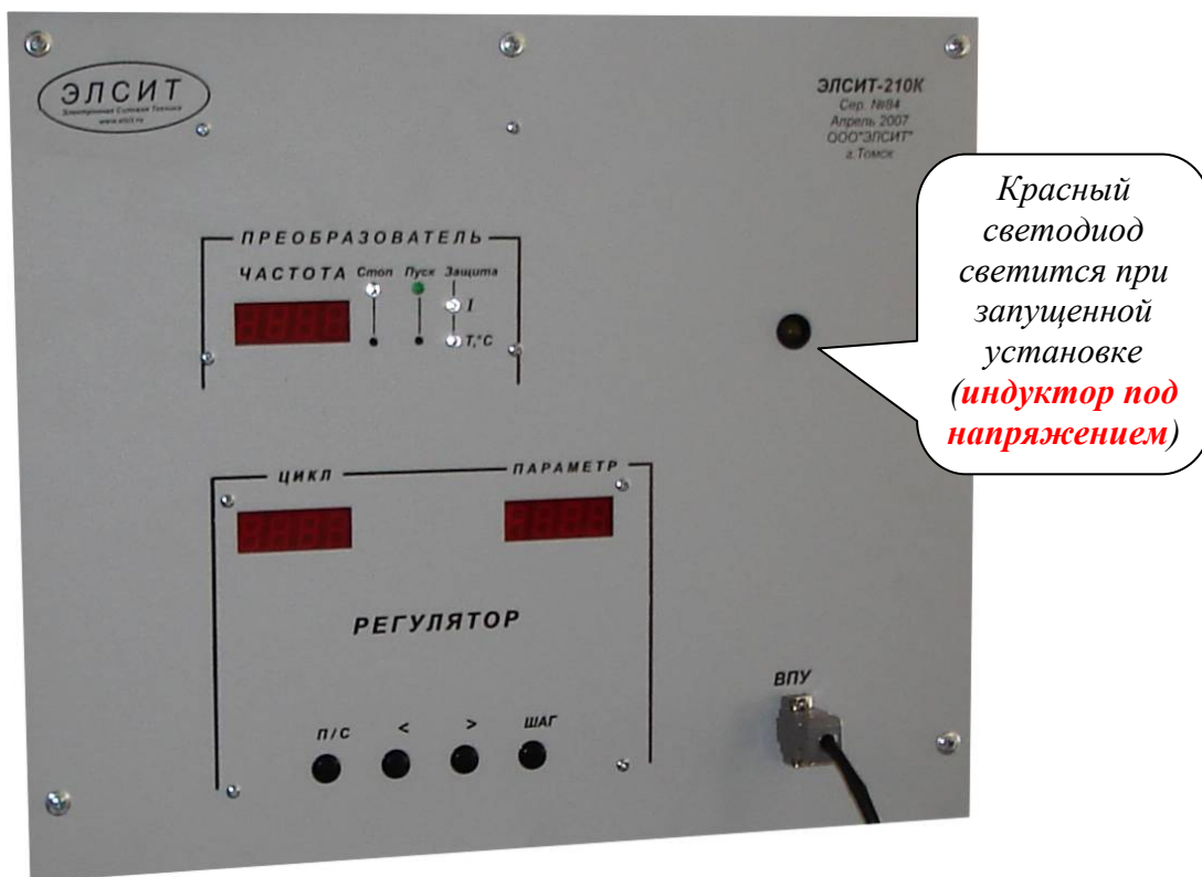
Рисунок 3. Передняя панель блока преобразователя.
