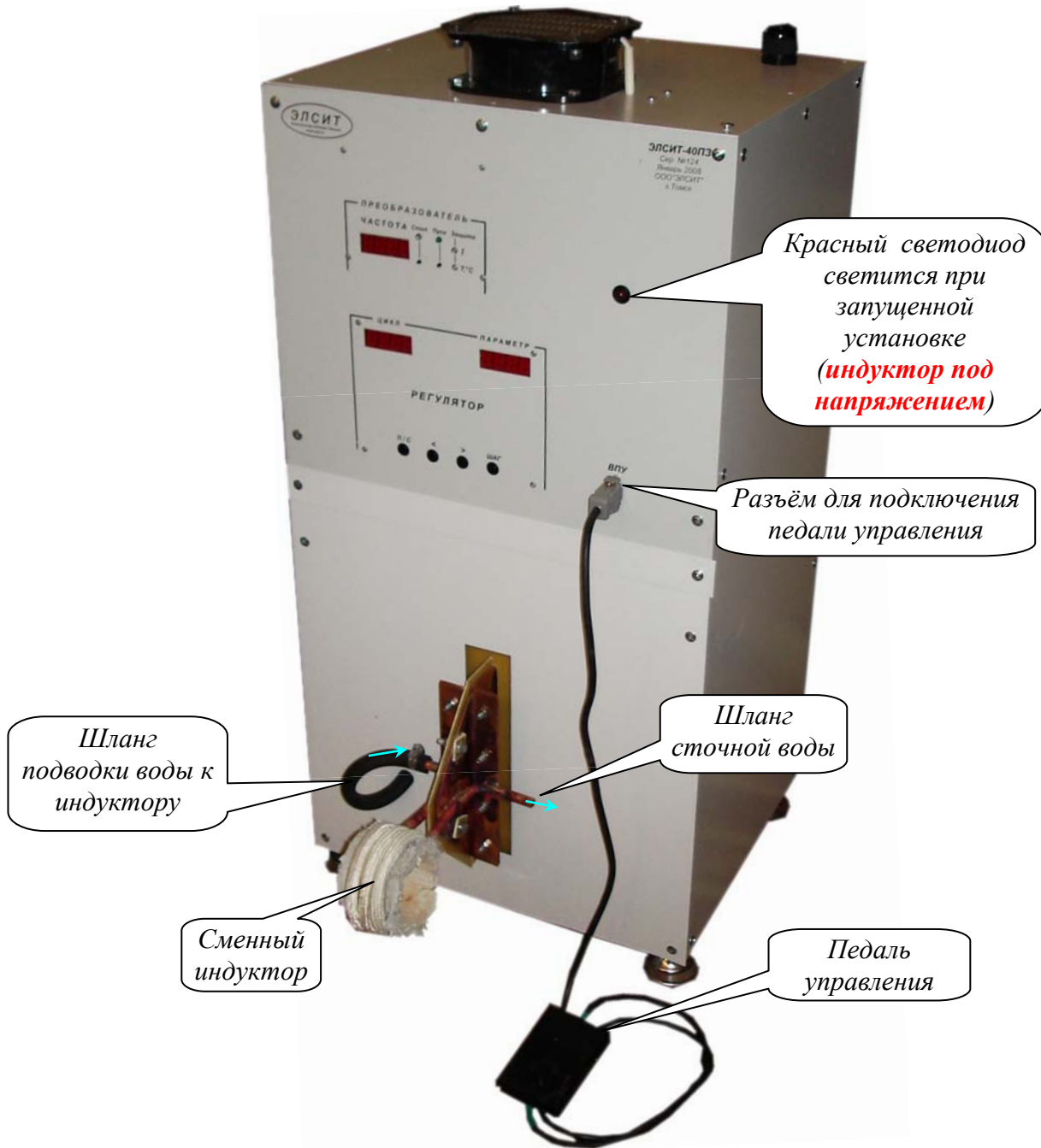
Рисунок 1. Силовой блок преобразователя (лицевая панель)
