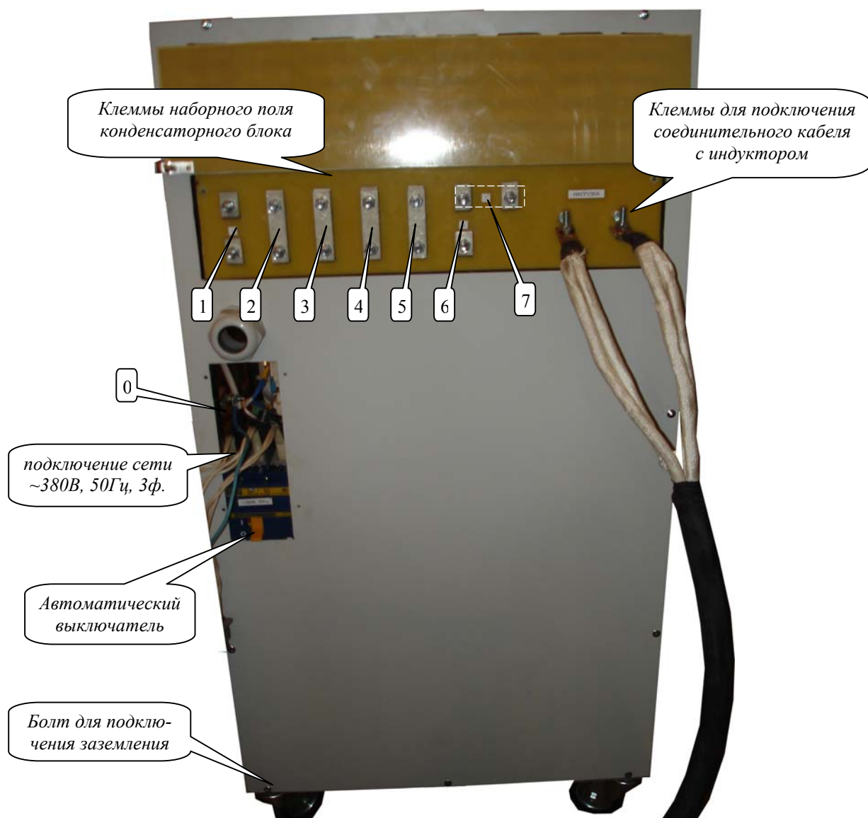
Рисунок 3. Задняя панель СП
