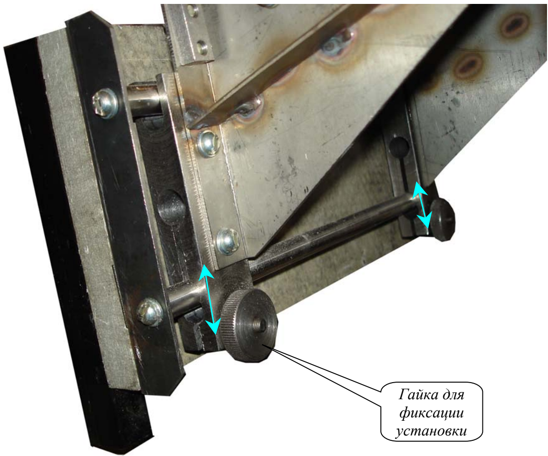
Рисунок 3 – Настройка подачи под разные диаметры.
