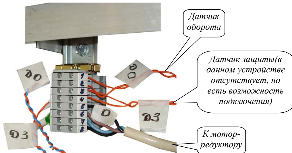
Рисунок 3 – Подключение устройства подачи.
